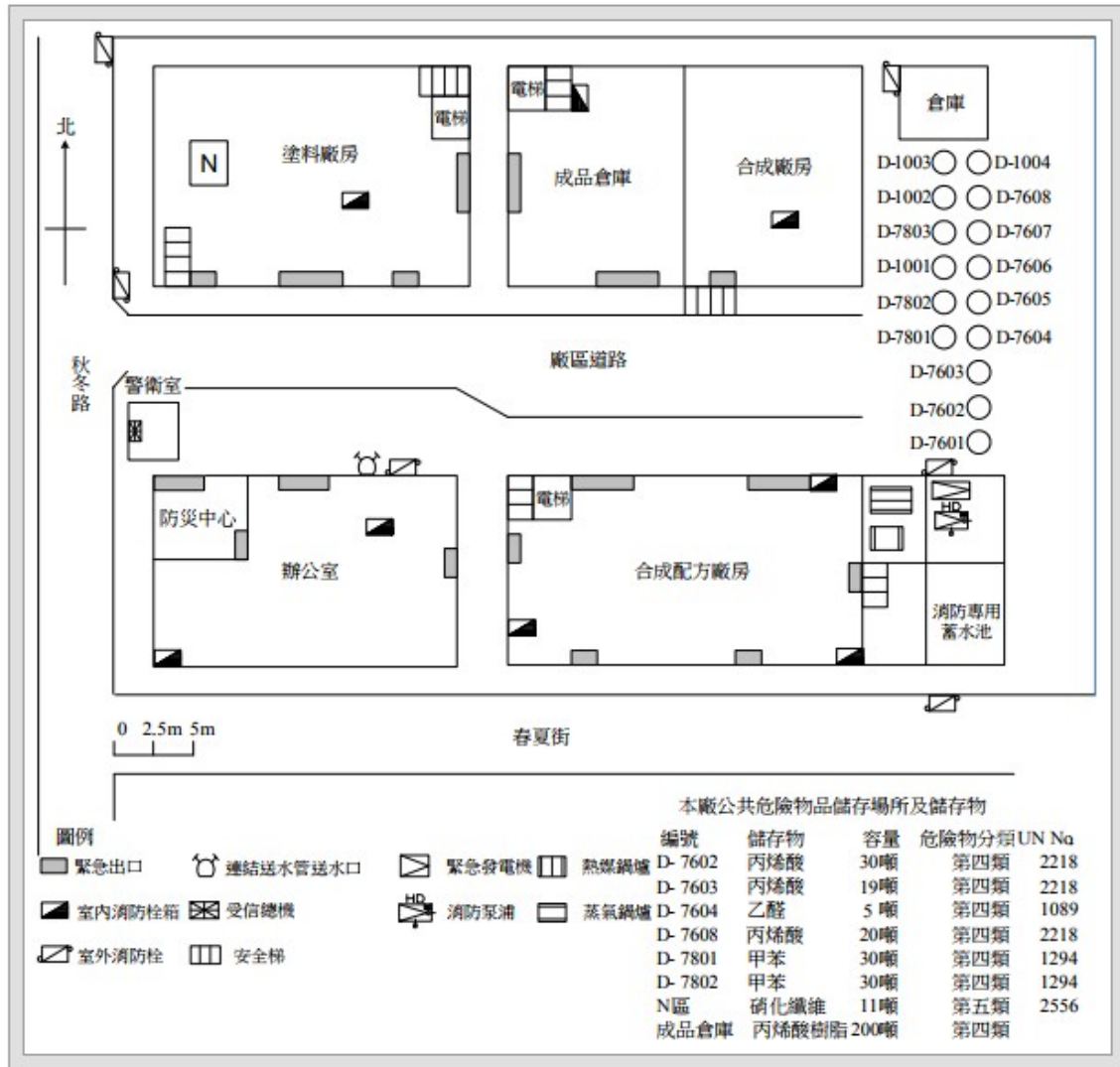
附件 18 廠區平面配置圖
